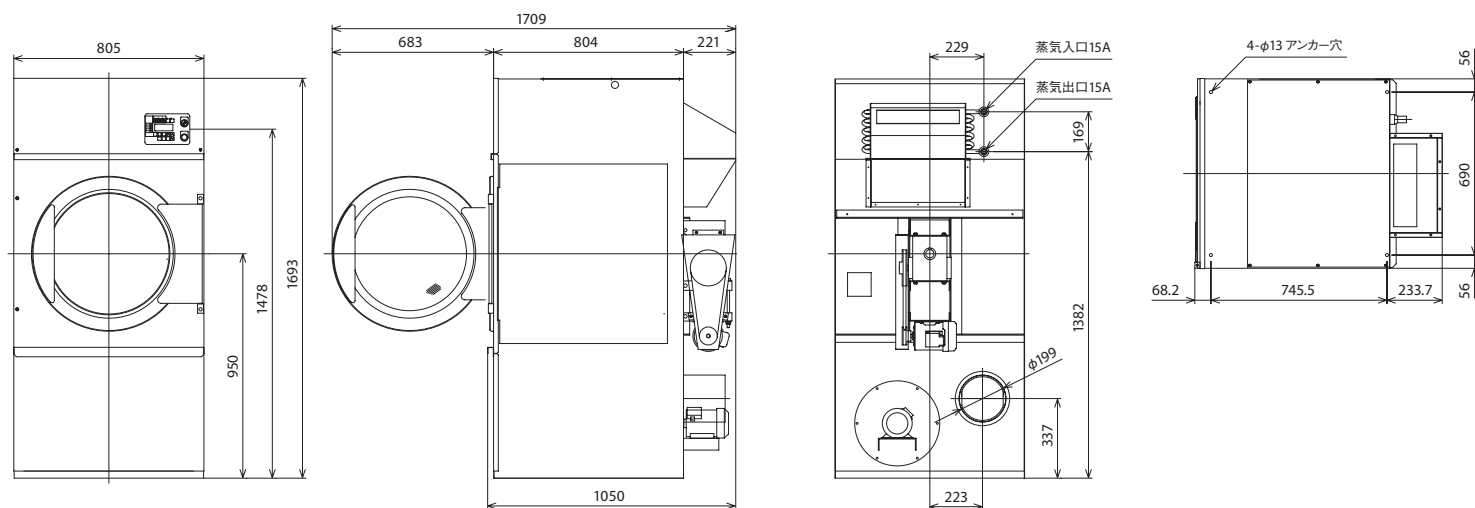
*図はTD-1303SM
